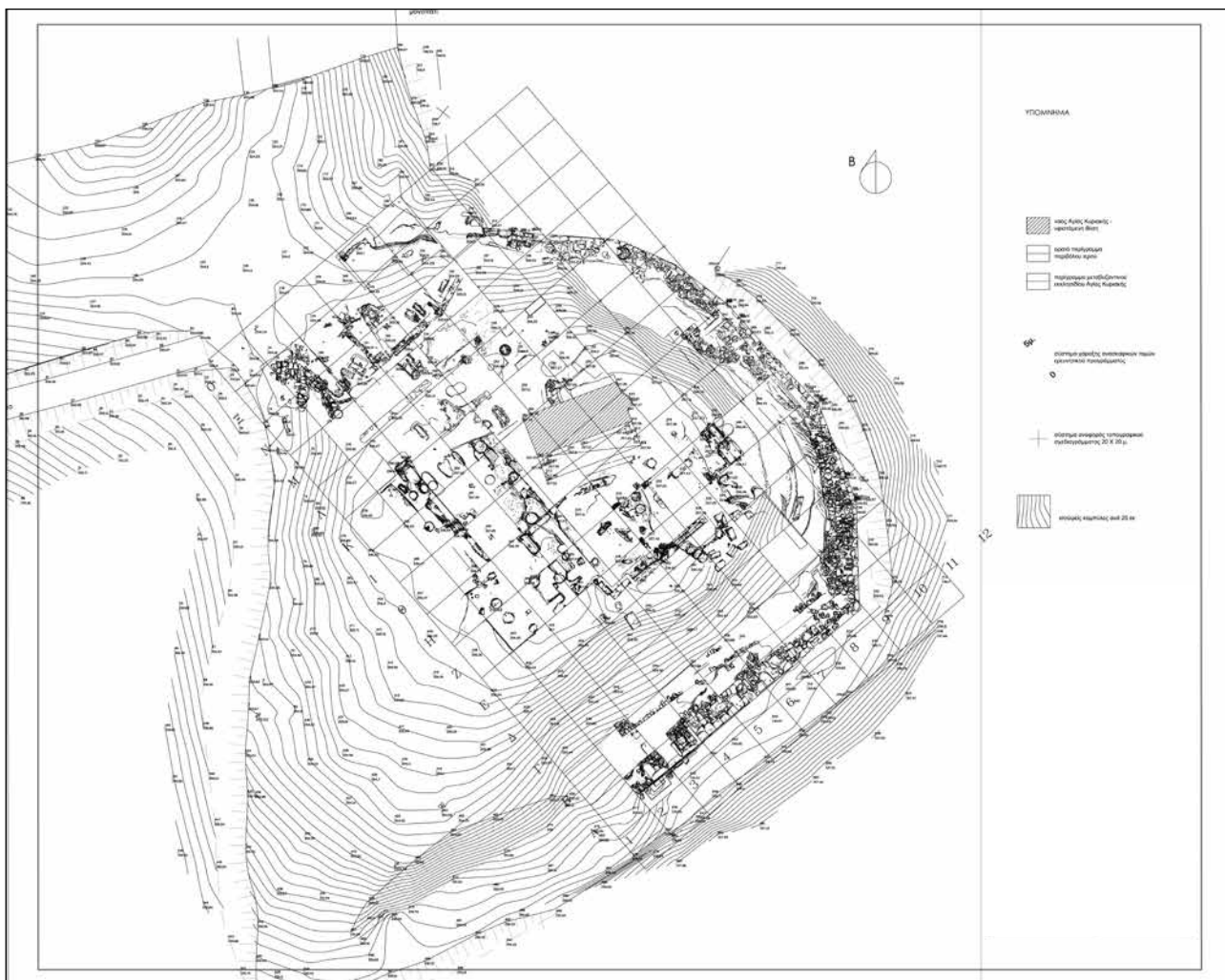
Εικ. 104. Αμύκλες. Ιερό Αμυκλαίου Απόλλωνος. Σχεδιαστική αποτύπωση μετά τις εργασίες του 2013 (σχέδ. Θ. Μπιλής, Μ. Μαγνήσαλη).
